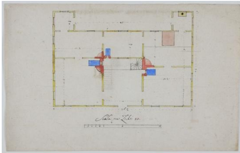
Ilustracja. Dwór drewniany do nieokreślonej miejscowości – projekt. Rzut przyziemia. Tylman van Gameren (1632-1706), Gabinet Rycin Biblioteki Uniwersyteckiej w Warszawie. 12
